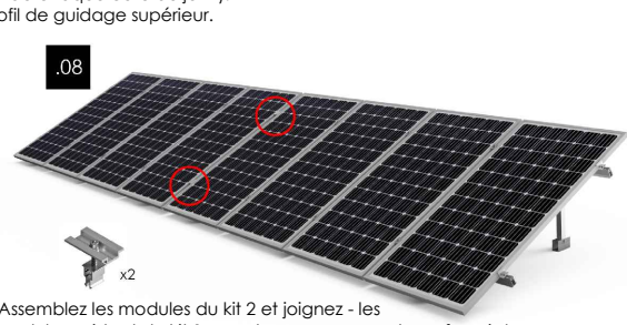
Kit 2 - Assemblez la structure de kit 2 et joignez au kit 1
