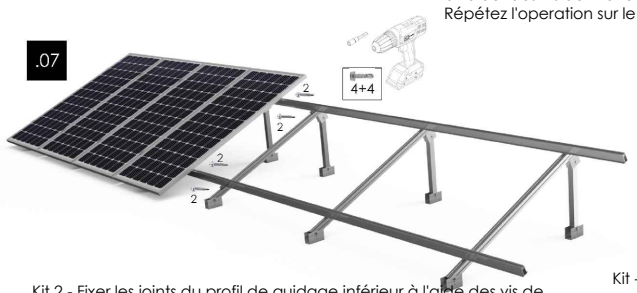
Kit 2 - Fixer les joints du profil de guidage inférieur à l'aide des vis de fixation (2 de chaque côté du joint) Répétez l'opération sur le profil de guidage supérieur.
