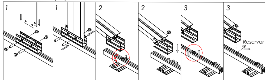
Apretar uniones
